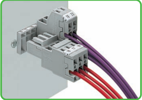
Монтажный блок и 1- и 2-проводные розетки
