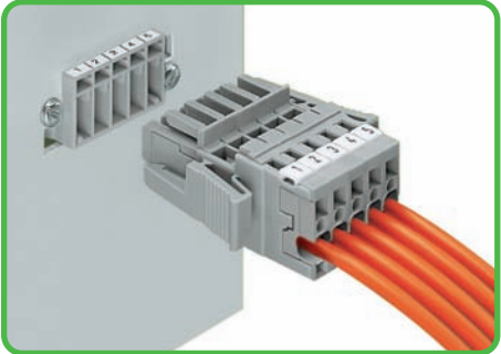
Монтажный блок и 1-проводная розетка с боковым фиксирующим рычагом
